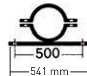
Rohrschelle 500 mm Lochabstand
