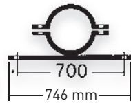
Rohrschelle 700 mm Lochabstand
