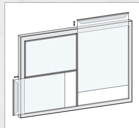
Profilsansicht Tiefe: 16 mm
