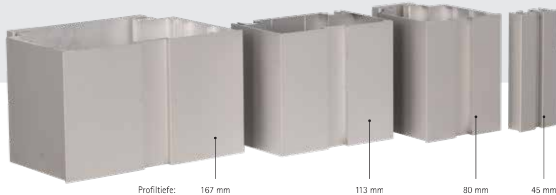
Seitenansicht unserer verschiedenen Profile (Bautiefen) unserer MADRID Außen- und Innenaufsteller.
